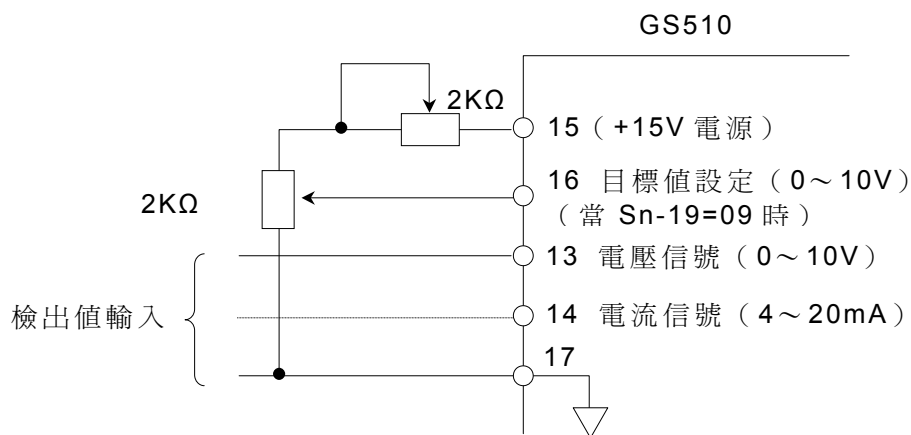
圖 11 PID 控制信號輸入
