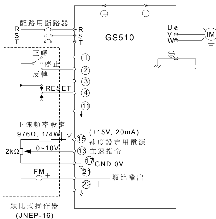
(b) 配線圖
