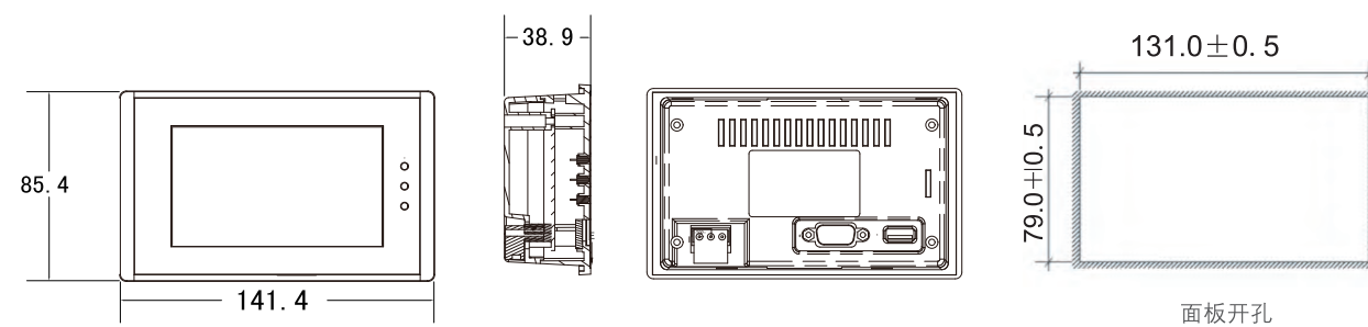
430L安装尺寸图
