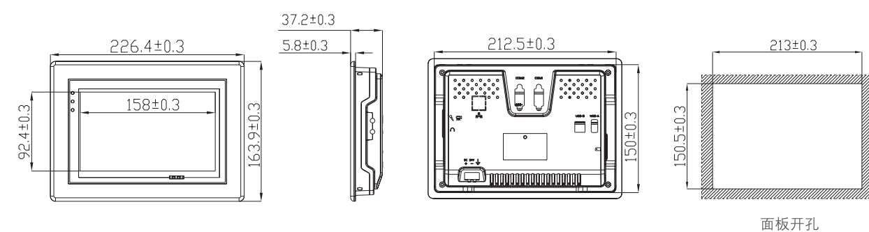
700A安装尺寸图
