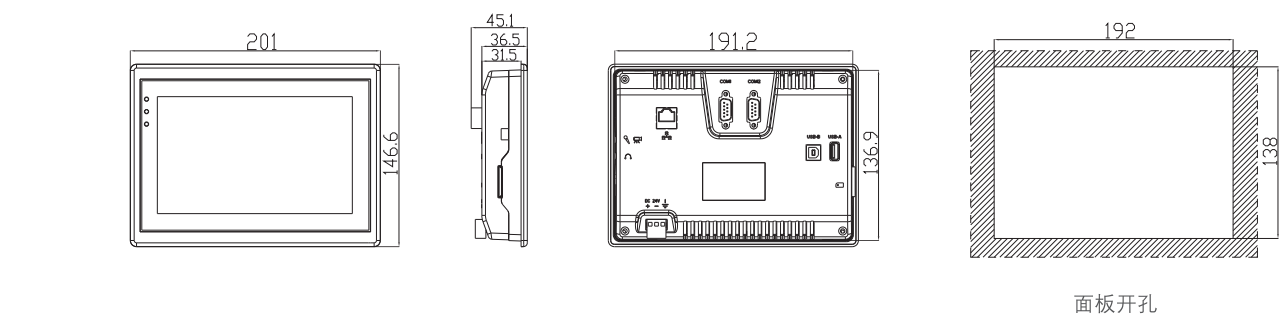
102A安装尺寸图
