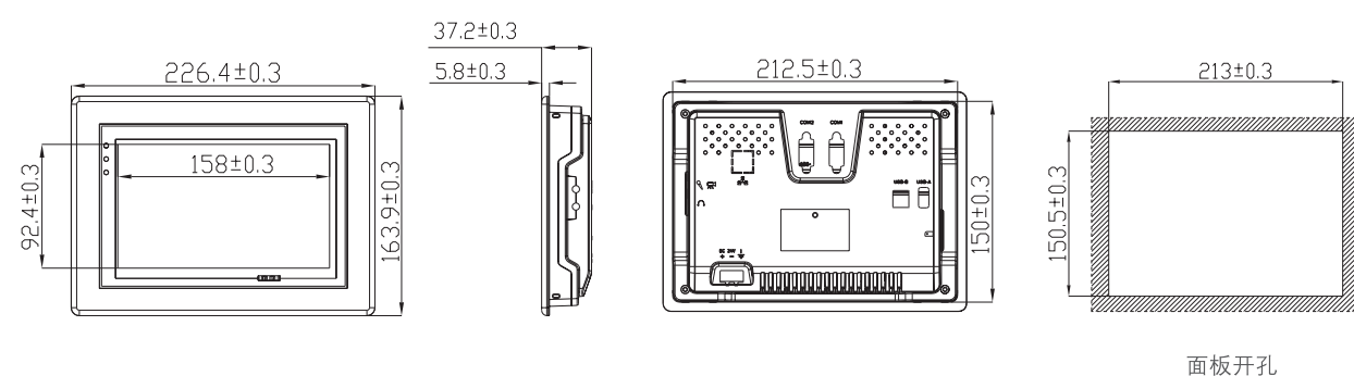
700L安装尺寸图
